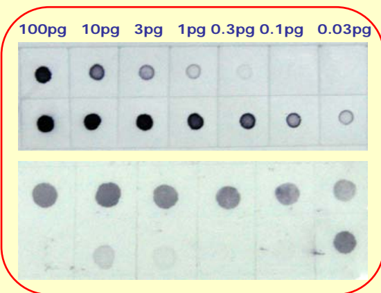
消减杂交阳性克隆 PCR 产物的反向 Northern 鉴定
